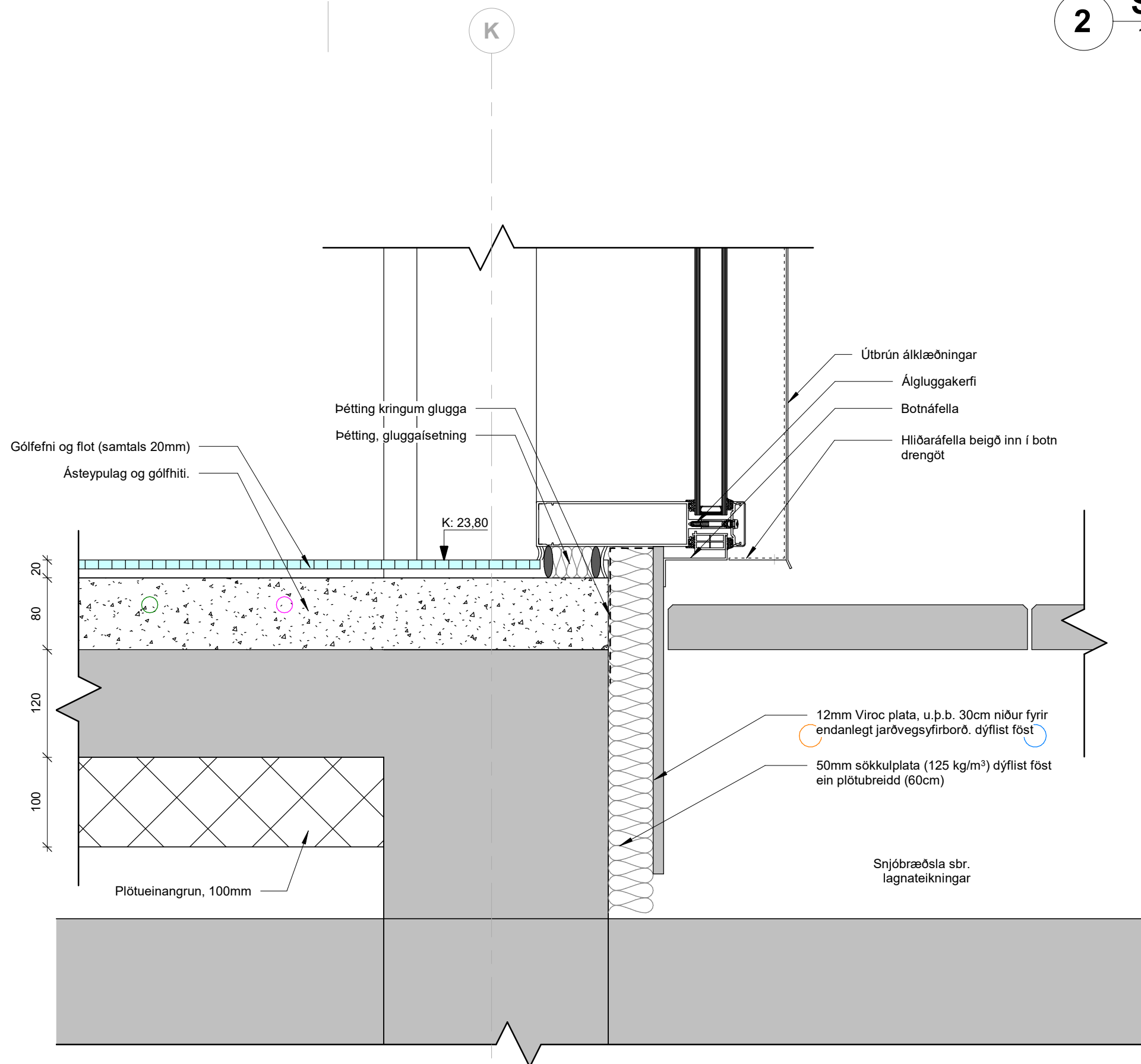
3 Sökkull, álgluggi 1 : 5
