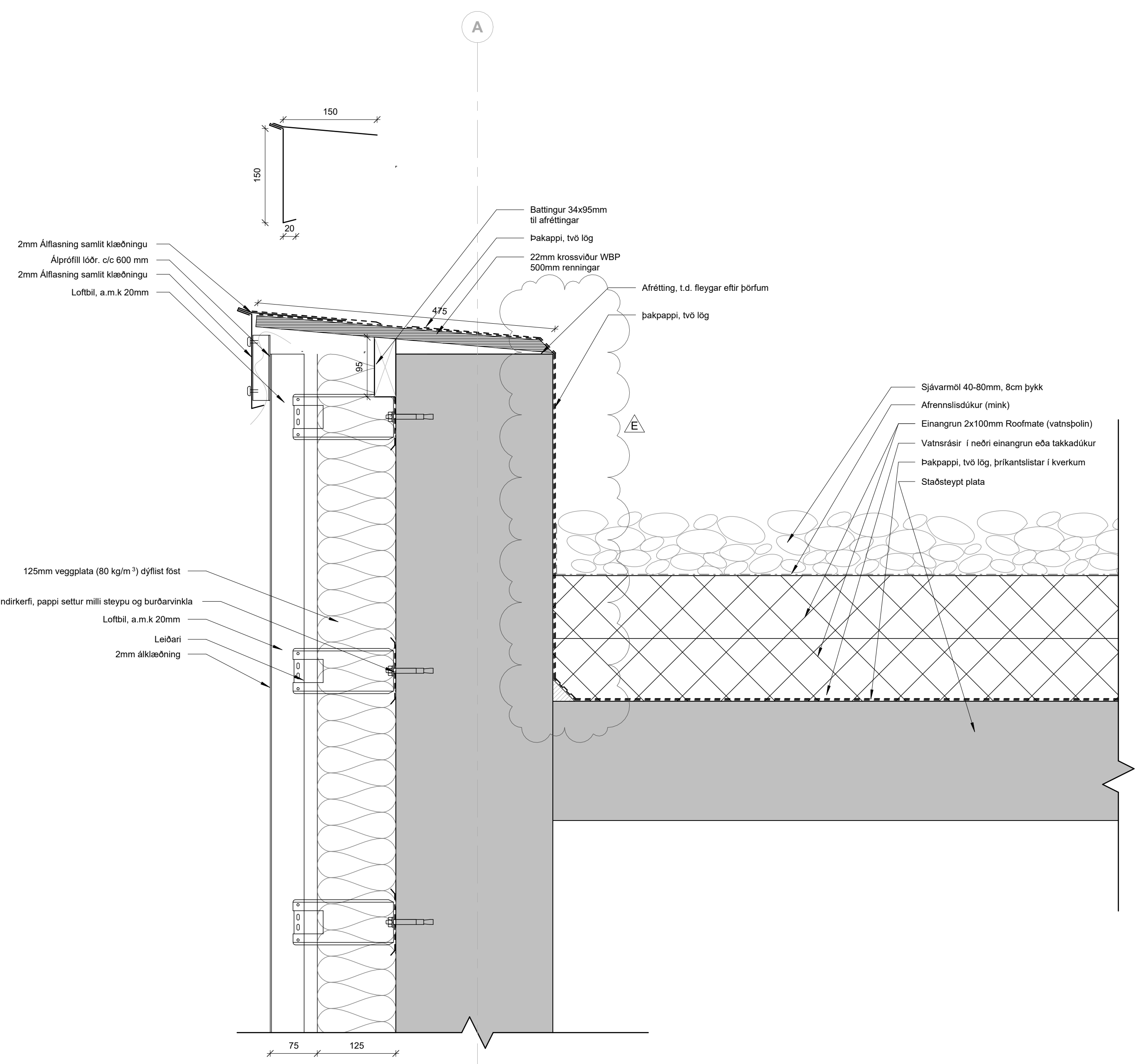
1 Viðsnúid þak, þakkantur 1 : 5
