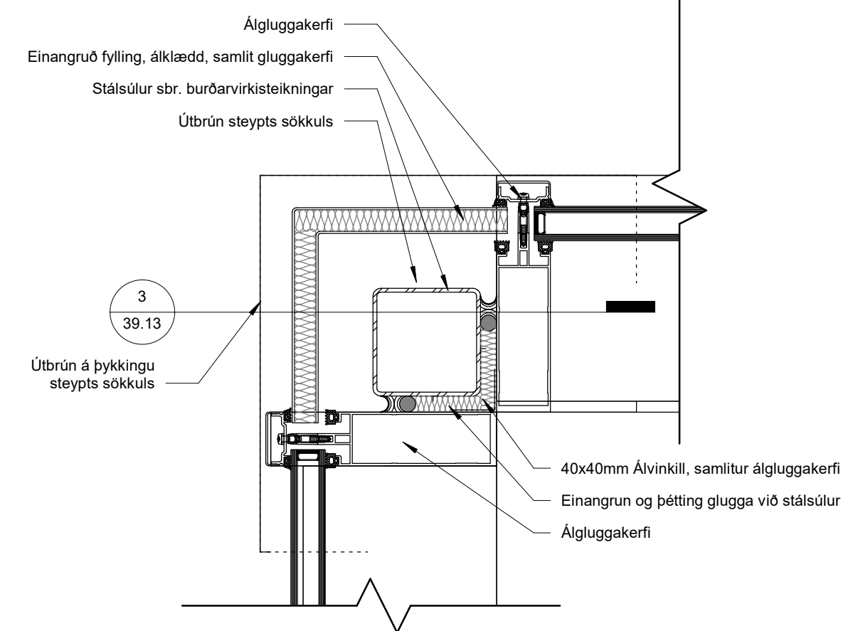
2 Vindfang úthorn 1 : 5
