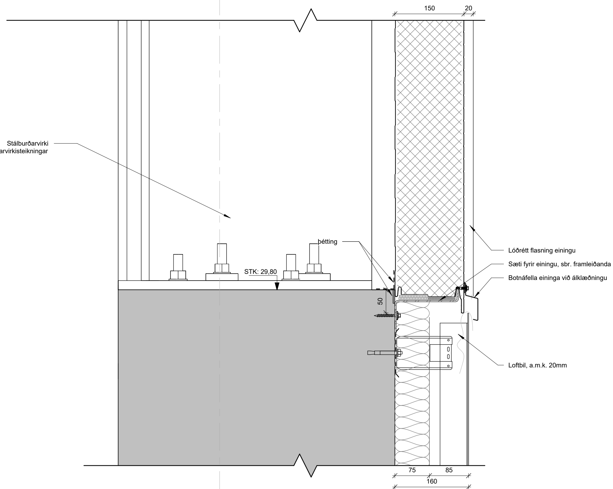
3 Steinullareiningar, við álklaðningu 1 : 5
