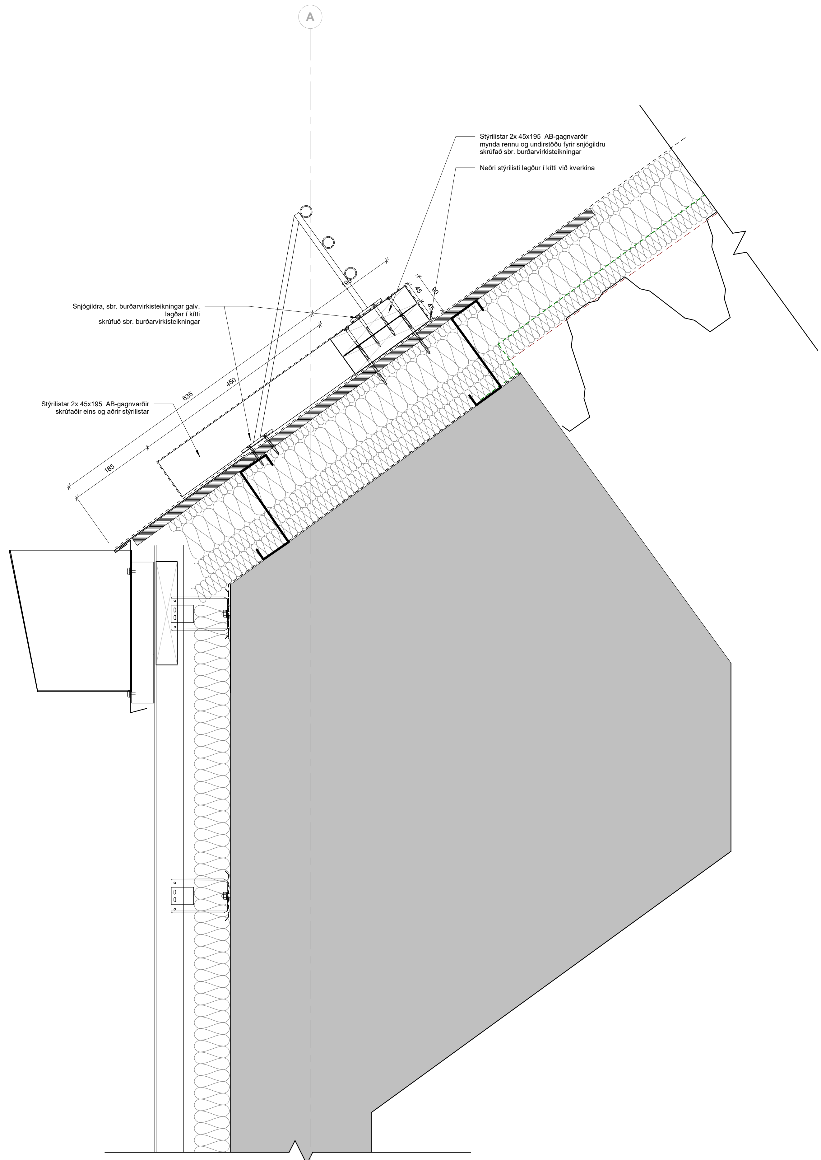
1 Stýrilistar og snjógildra neðri staða 1:5
