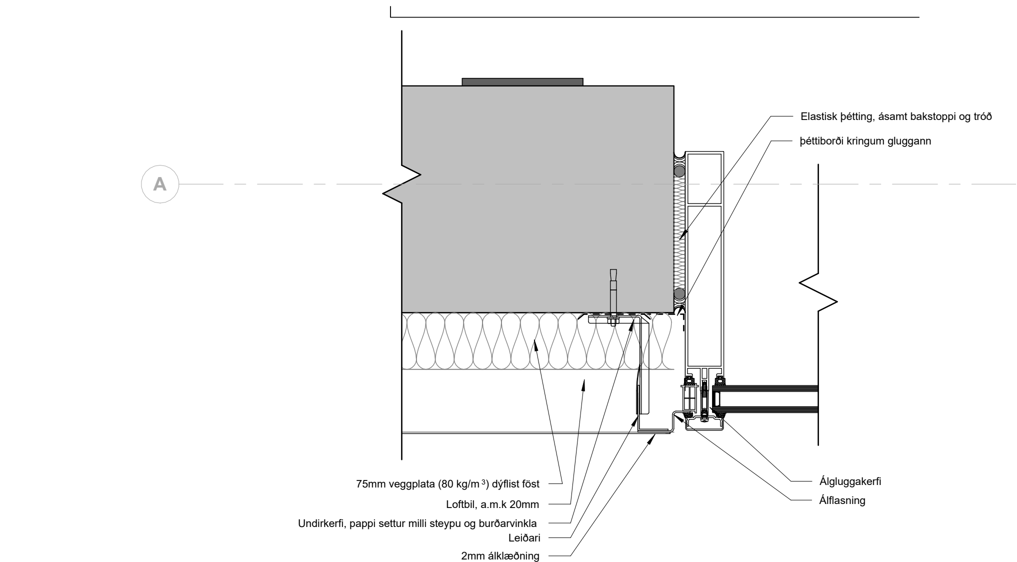
5 Álklæðning, salur, álgluggi, hlið 1:5
