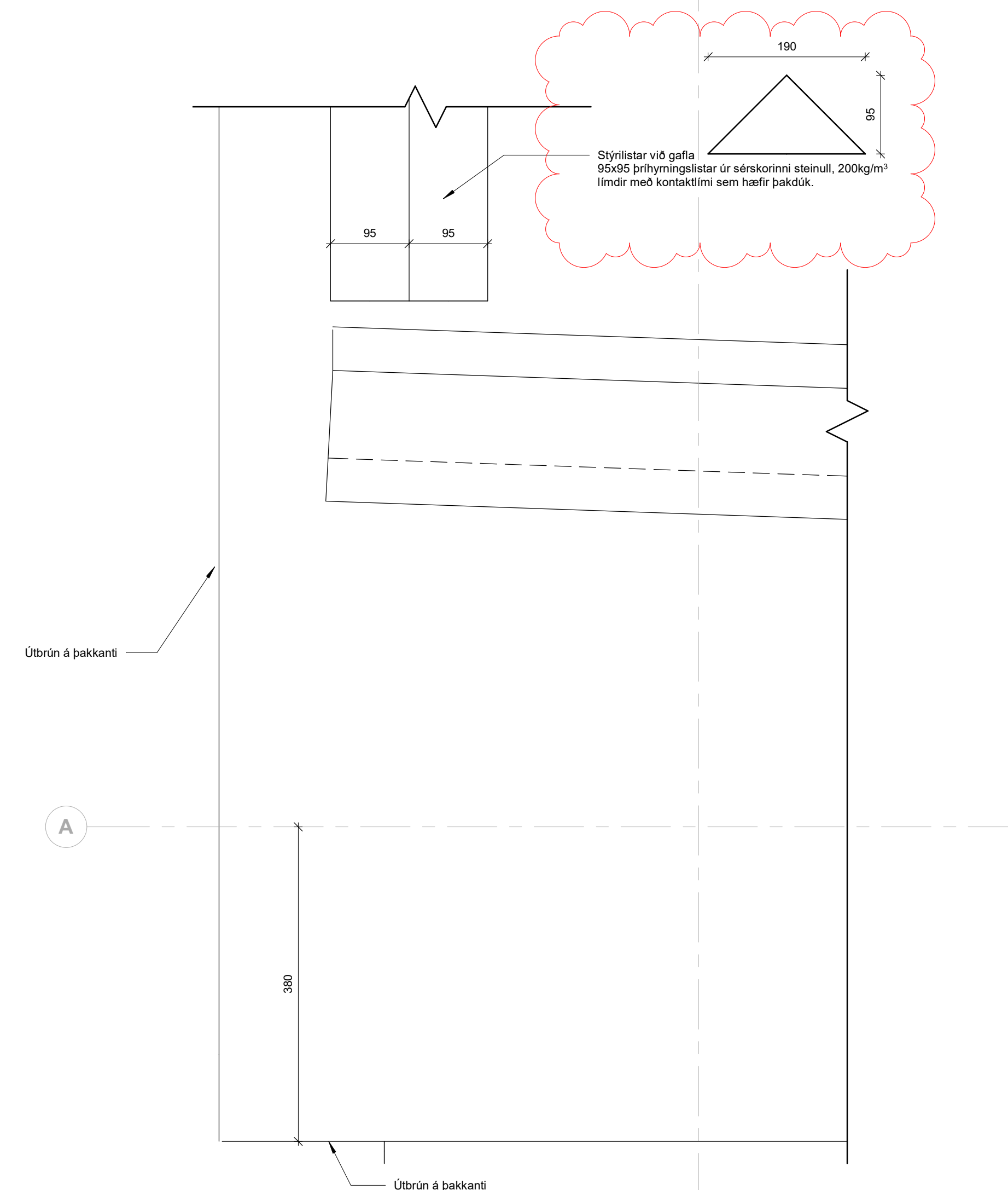
3 Listar að niðurfallstrektum, horn 1 : 5
