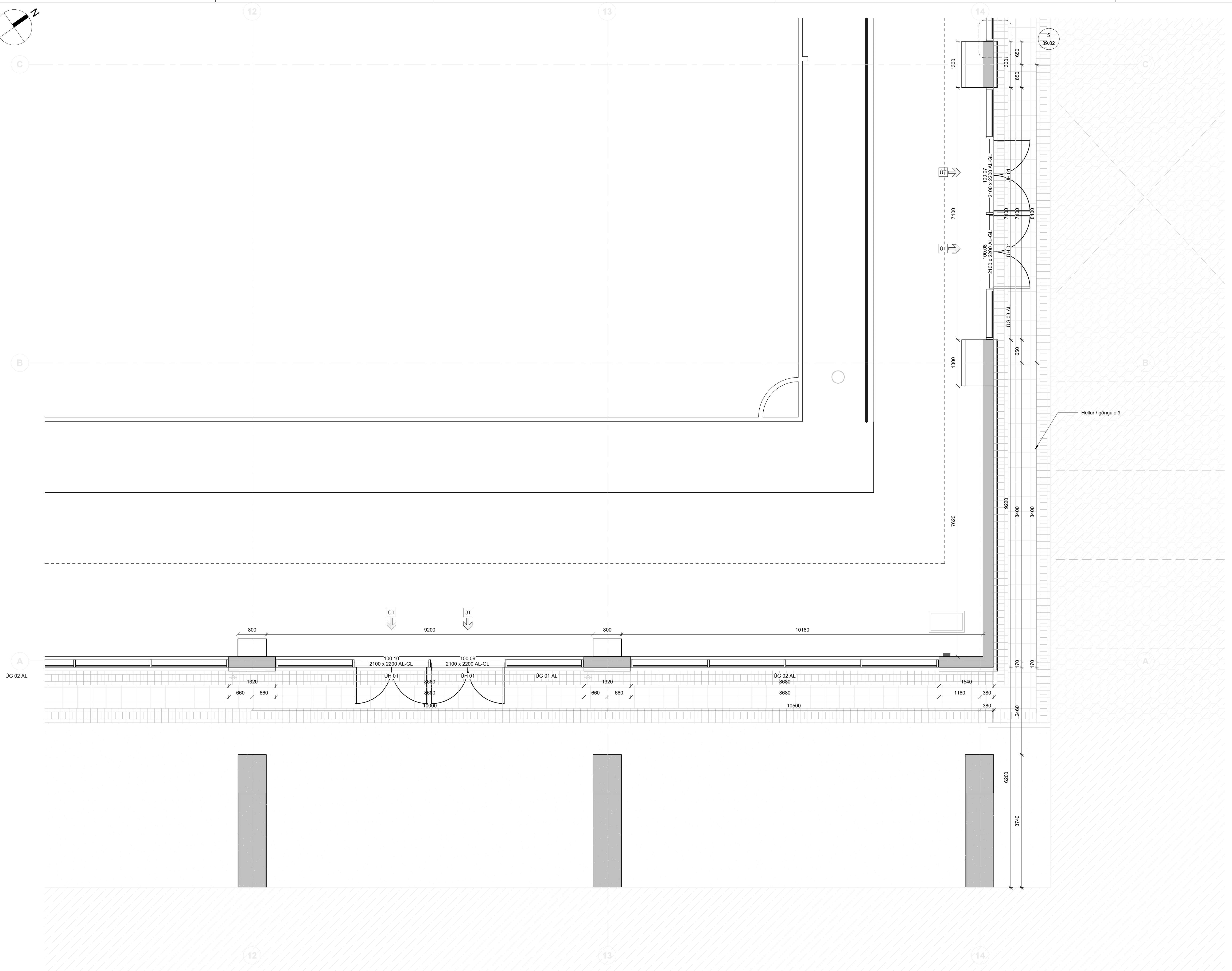
1. Hæð grmd - Svæði 164 1 : 50
