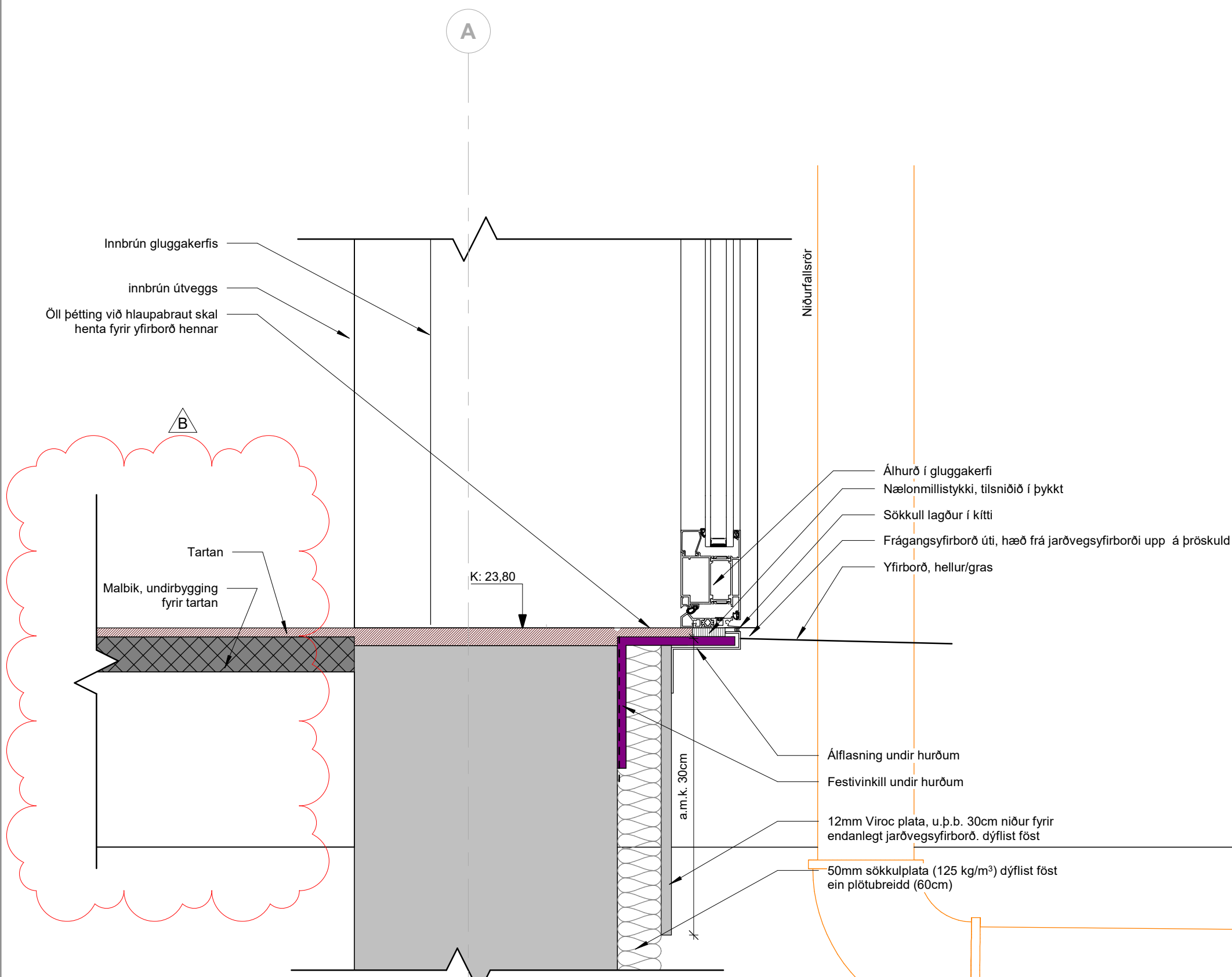
1 Sökkull, salur, álhurð 1 : 5
