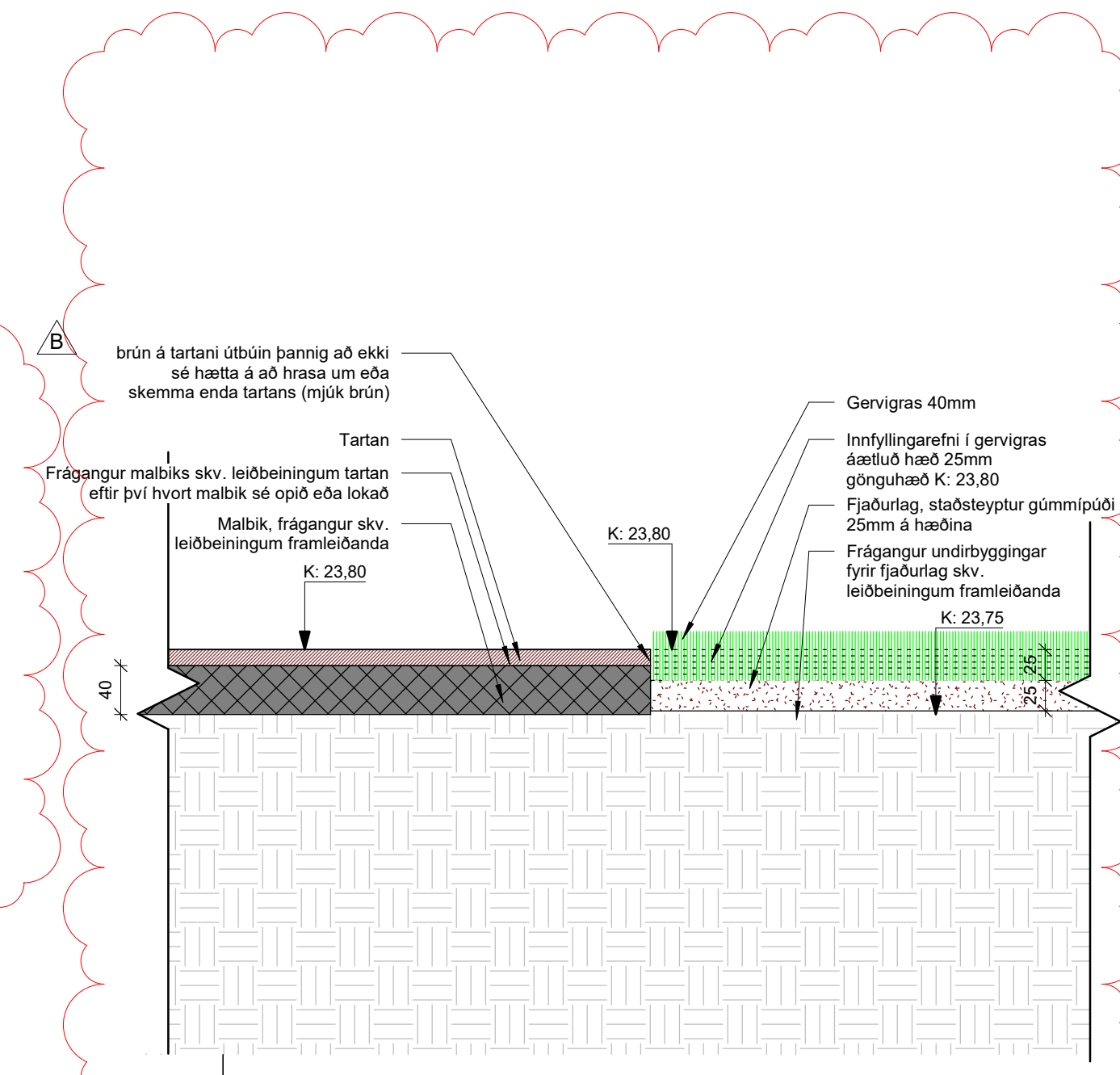
5 Hlaupabraut mætir gervigrasi 1 : 5
