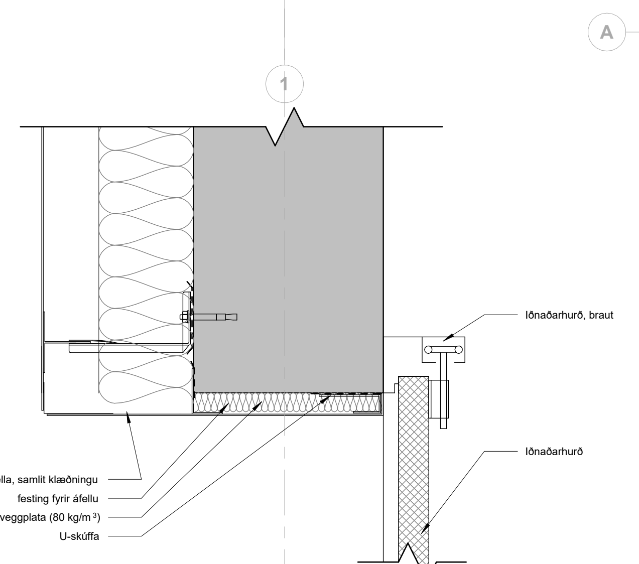
6 Álklæðning, iðnaðarhurð, hlið 1:5
