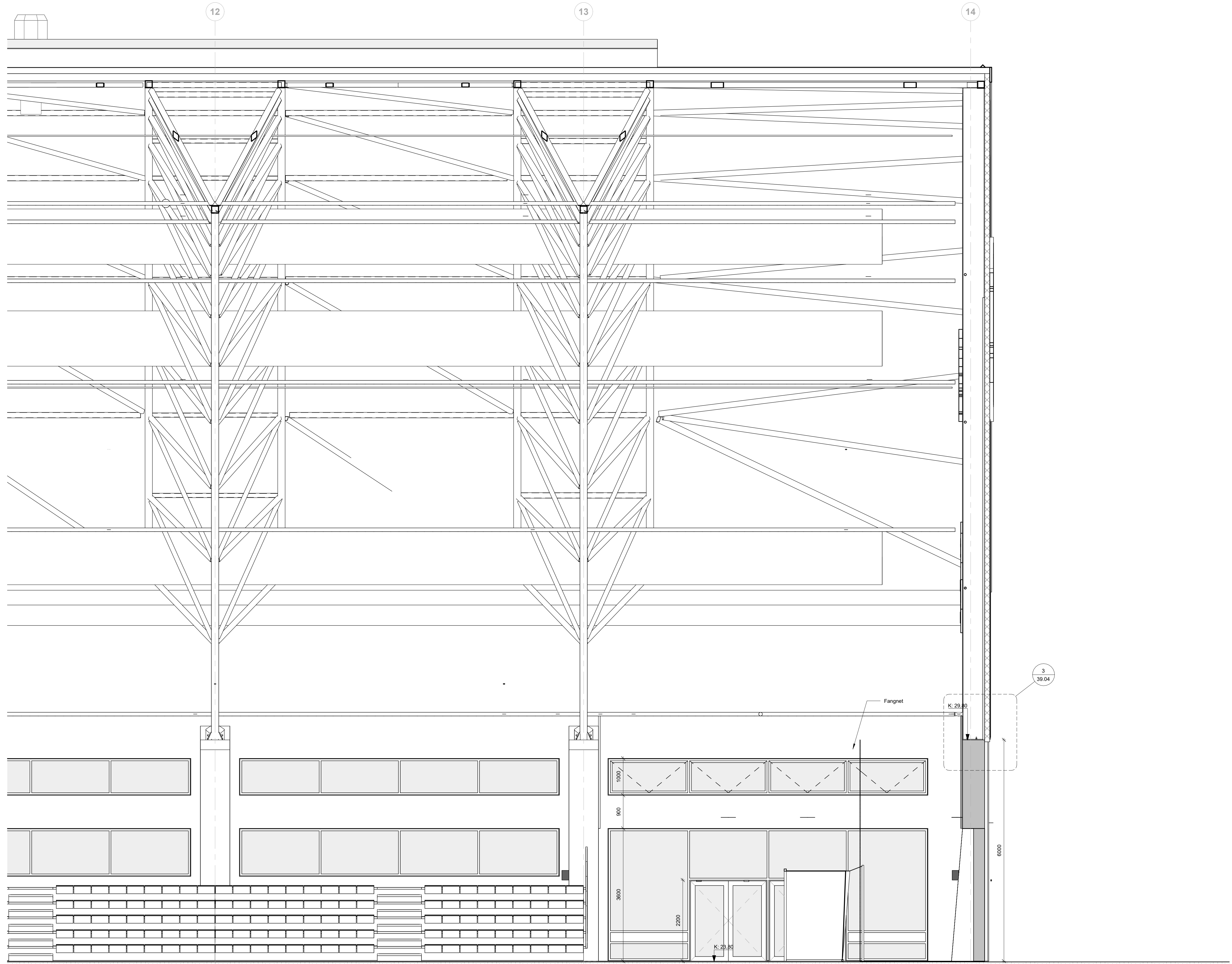
1 20-F-V - Hluti 6 1:50
