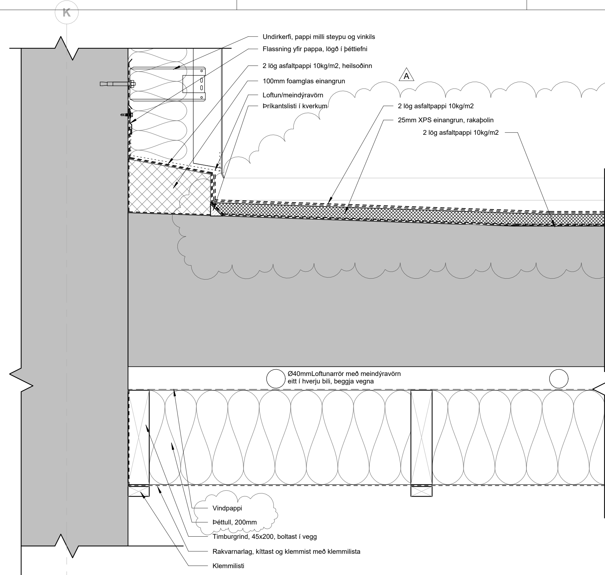
1 Þakskyggni við útvegg 1 : 5
