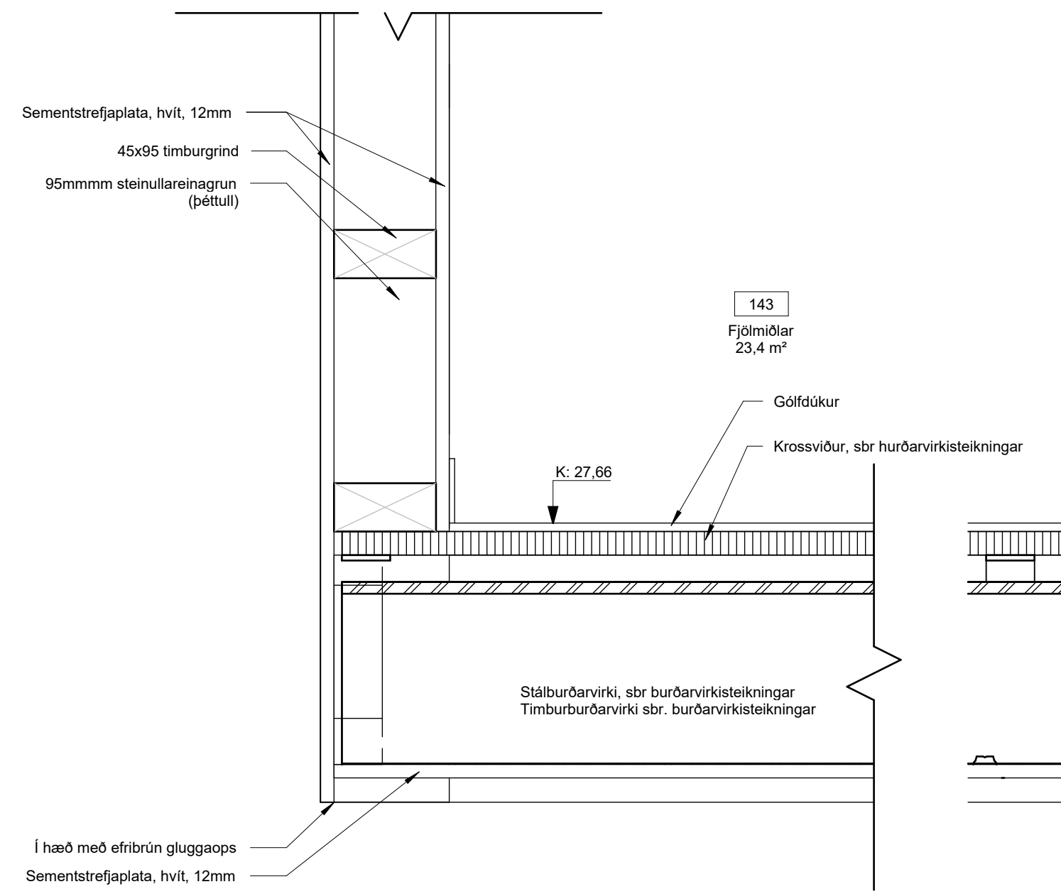
2 Gólf og veggir fjölmiðlapallur 1 : 5
