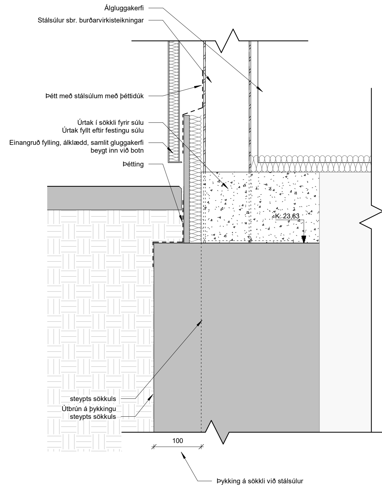
3 Frágangur við súlur í vindfangi 1 : 5
