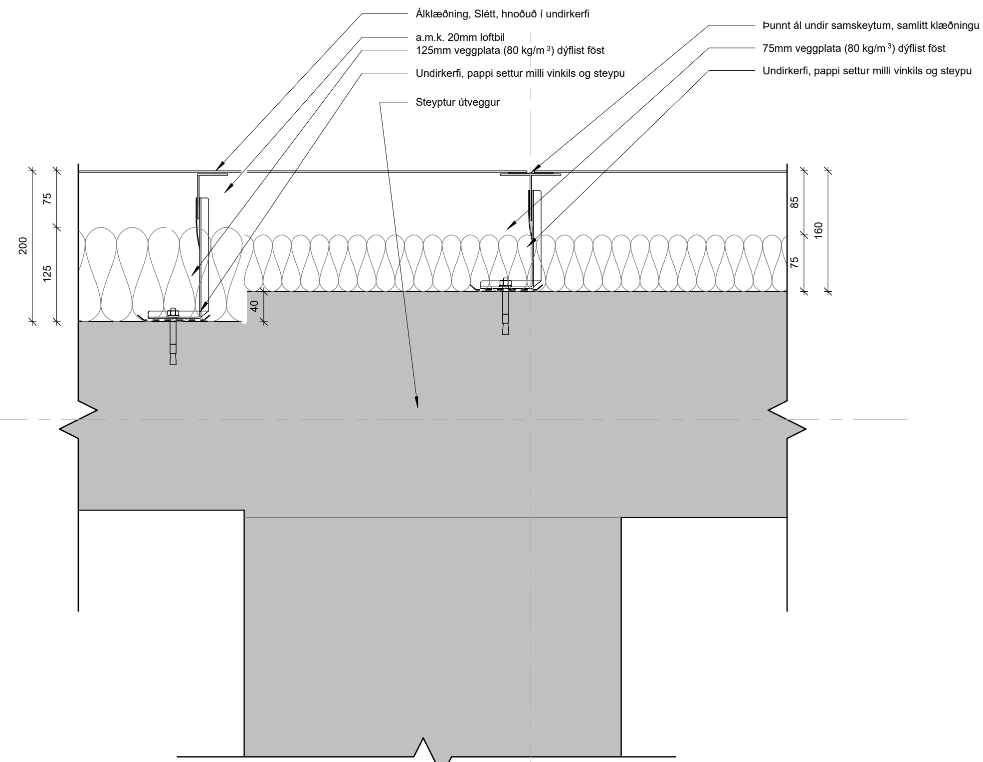
2 Álklæðning, við veggþykkingu 1:5
