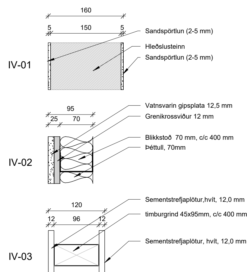
4 Léttir innveggir 1 : 5
