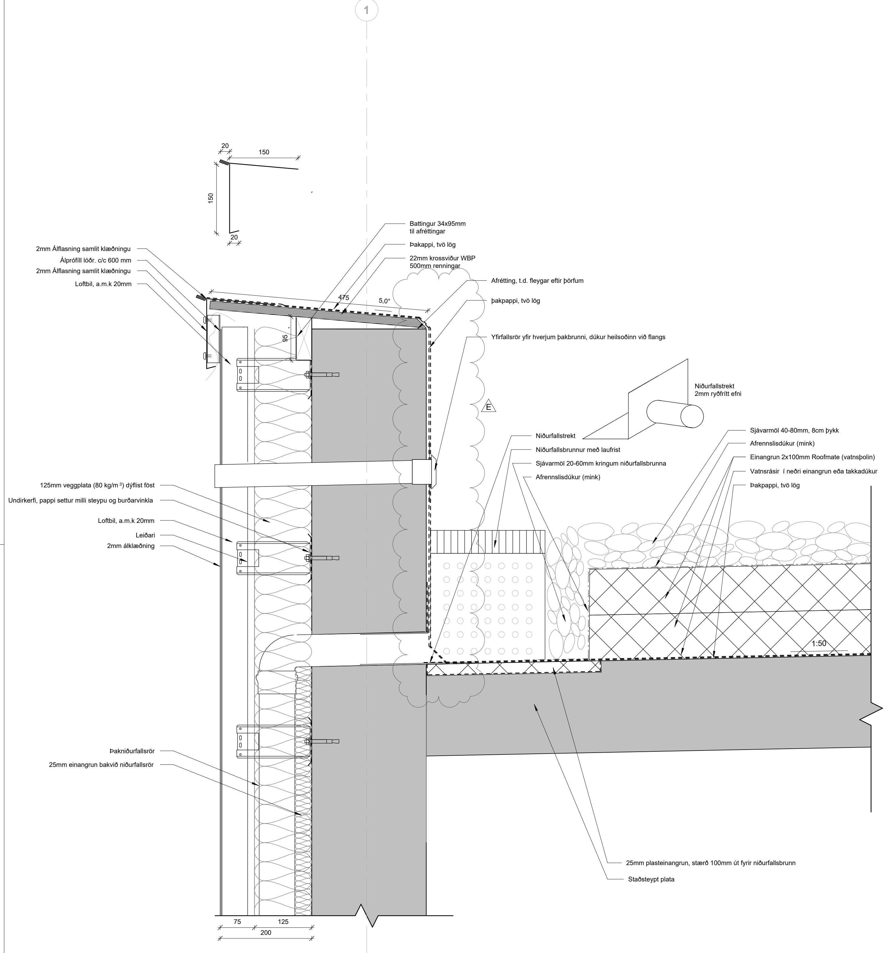
1 Viðsnúð þak, Þakbrunnur 1 : 5
