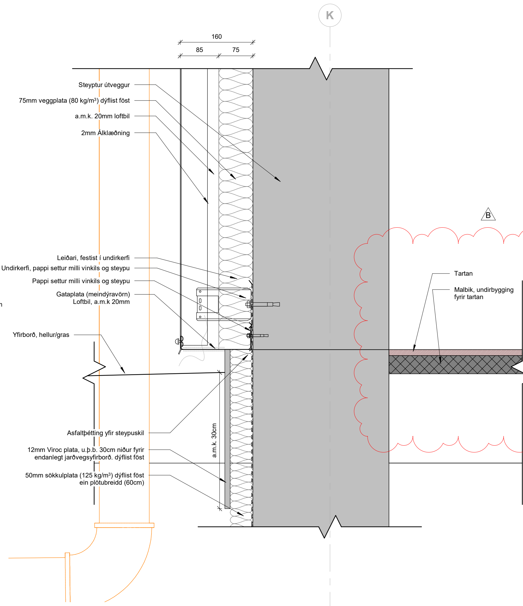
2 Sökkull, salur, álklaðning 1 : 5
