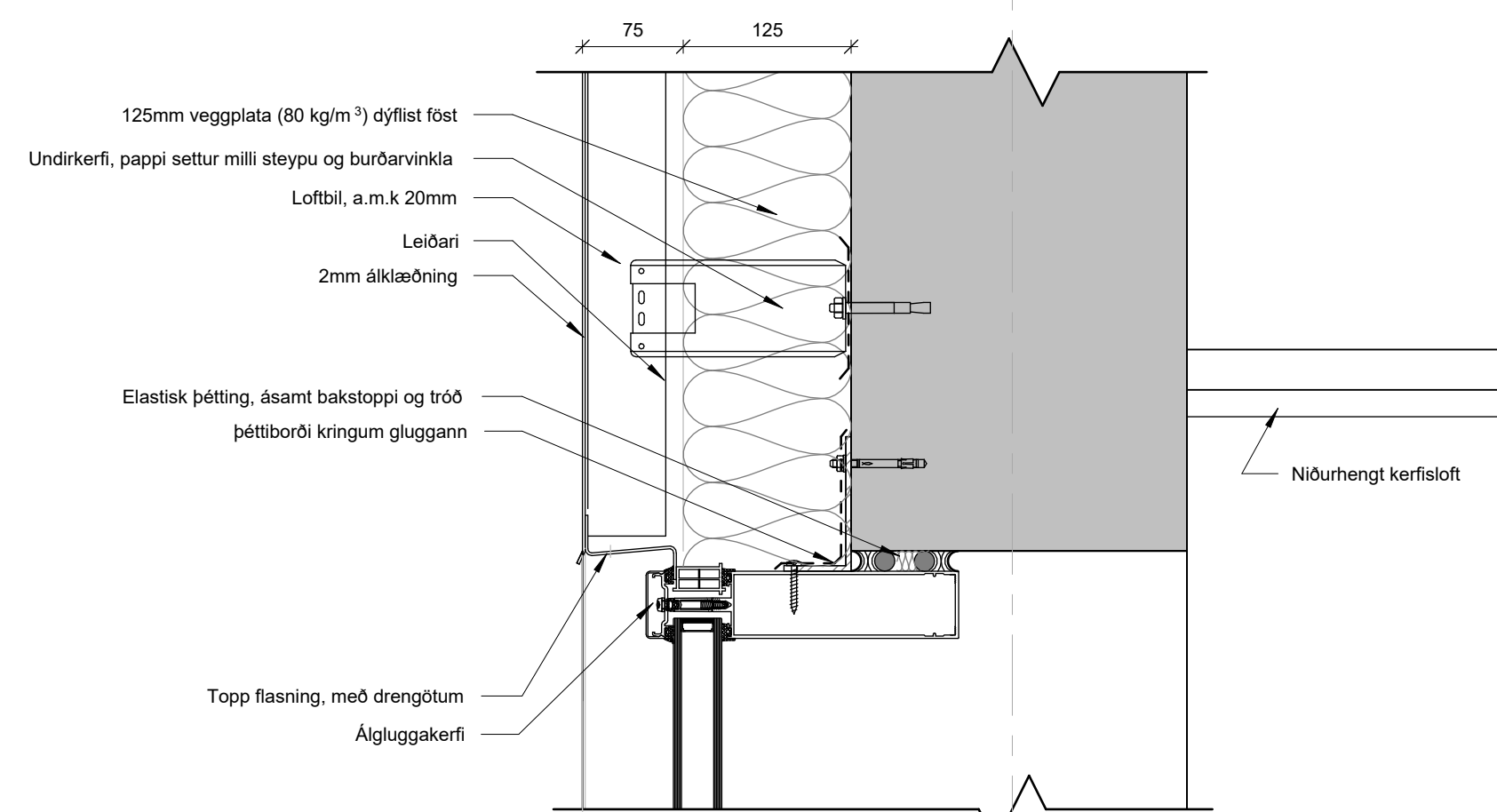
2 Álklaðning, álguggi, efri 1 : 5
