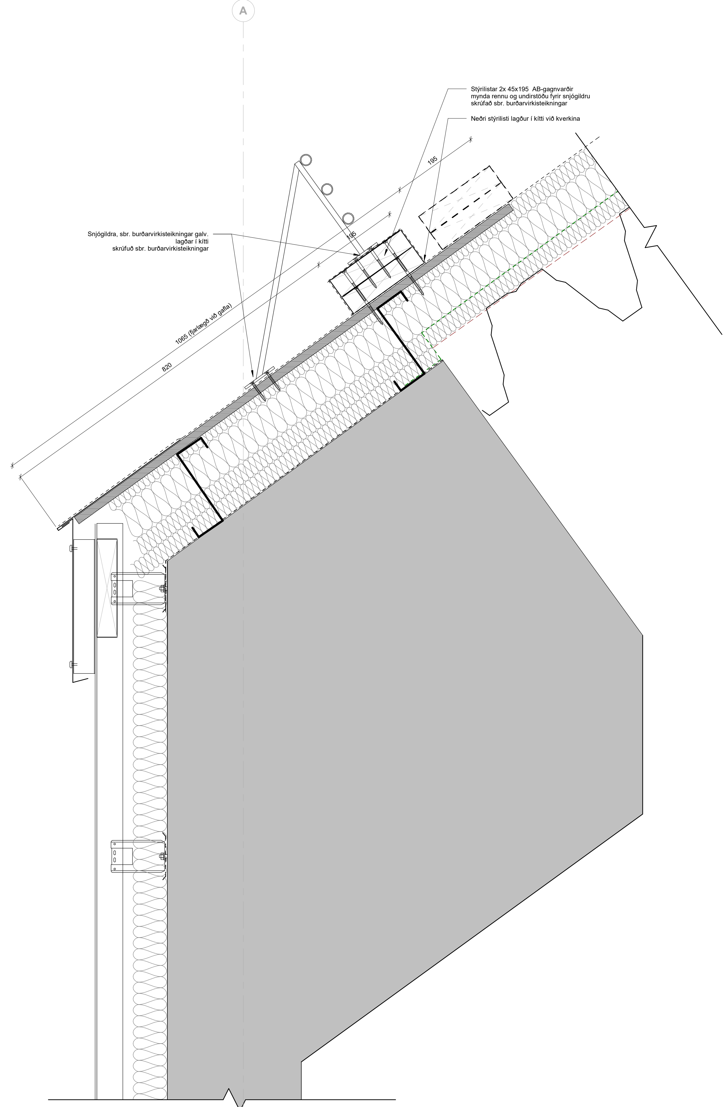
2 Stýrilistar og snjógildra efri staða 1:5
