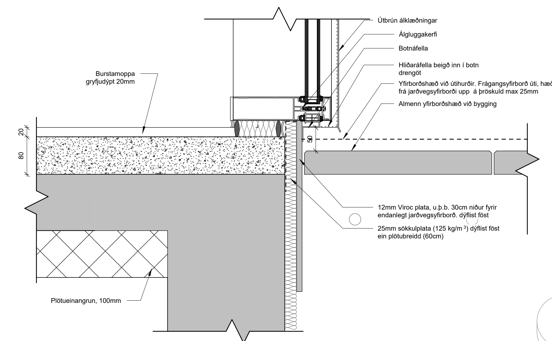
5 Sökkull við vindfang 1 : 5
