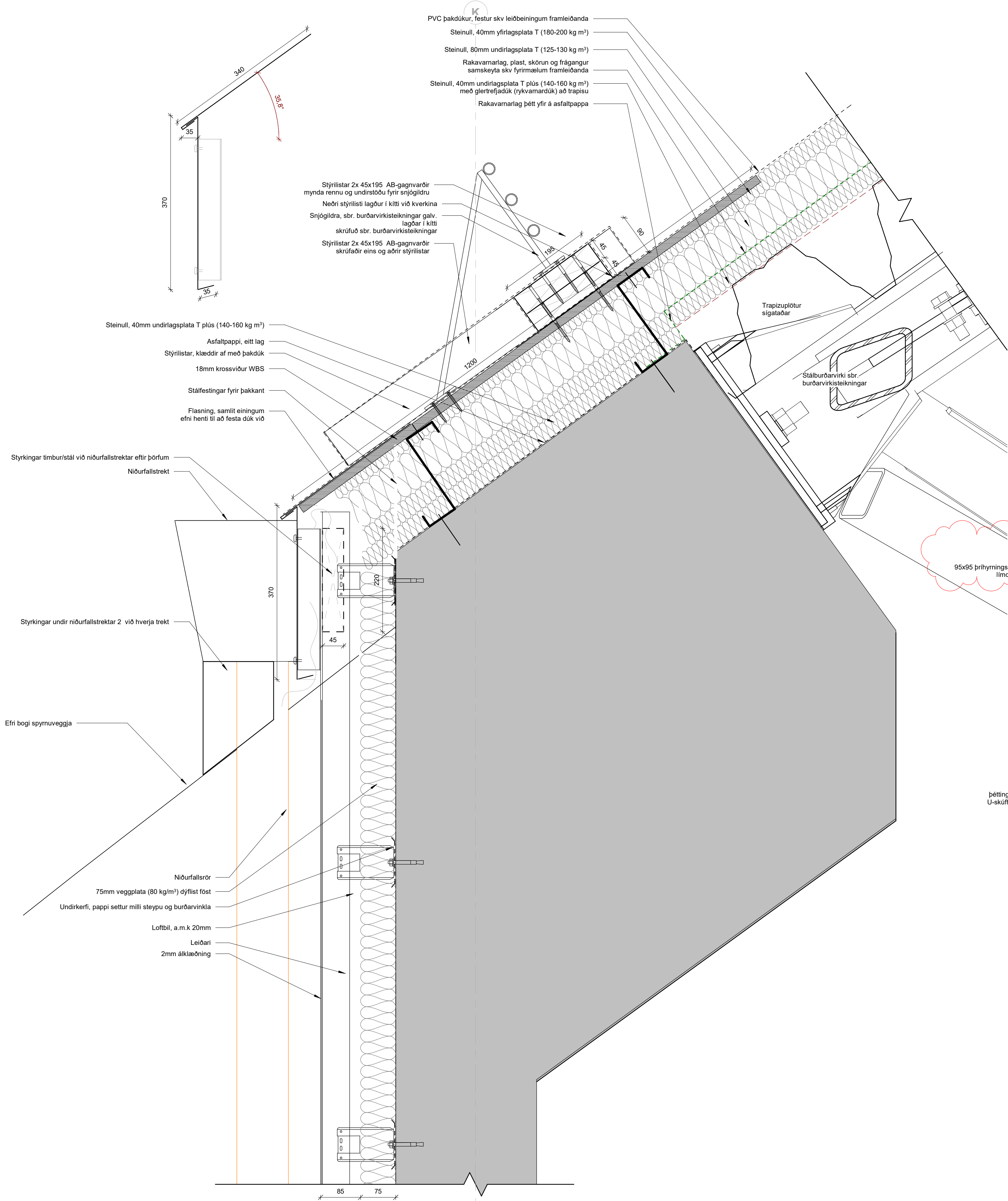
1 Þak, salur, neðri þakkantur 1 : 5
