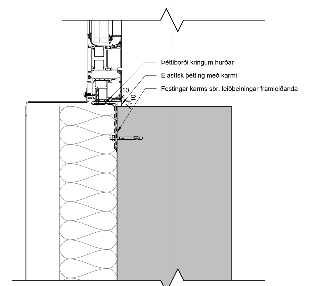
4 Álklæðning, álhurð, hlið 1:5
