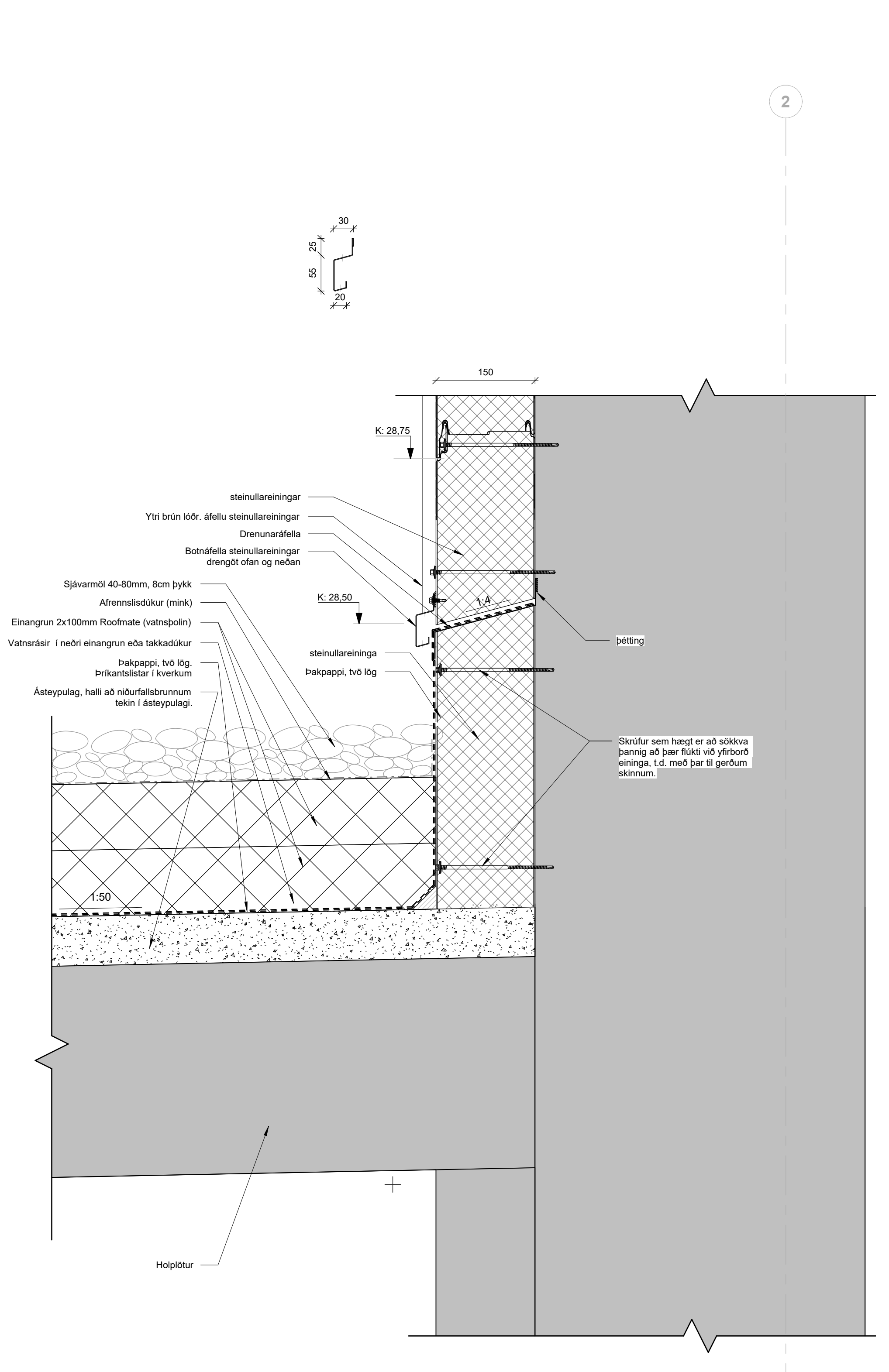
2 Viðsnúð þak, efri, holplötur 1 : 5
