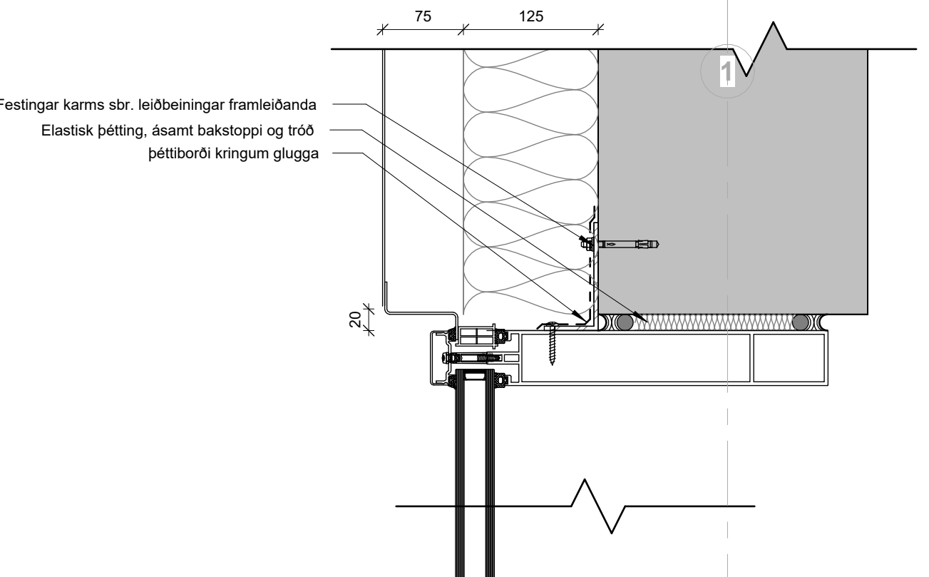
3 Álklæðning, álgluggi, hlið 1:5
