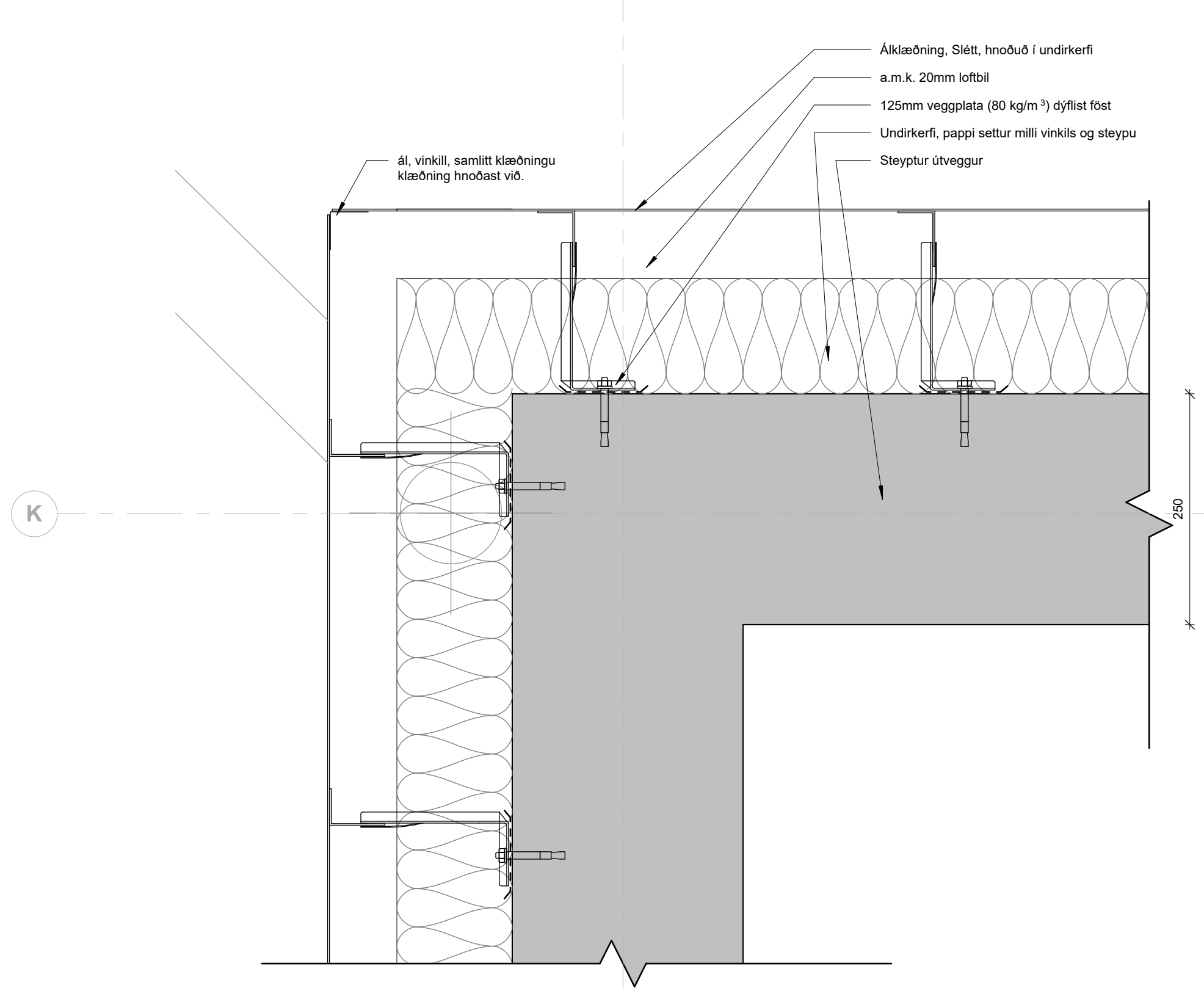
1 Álklæðning, úthorn 1:5
