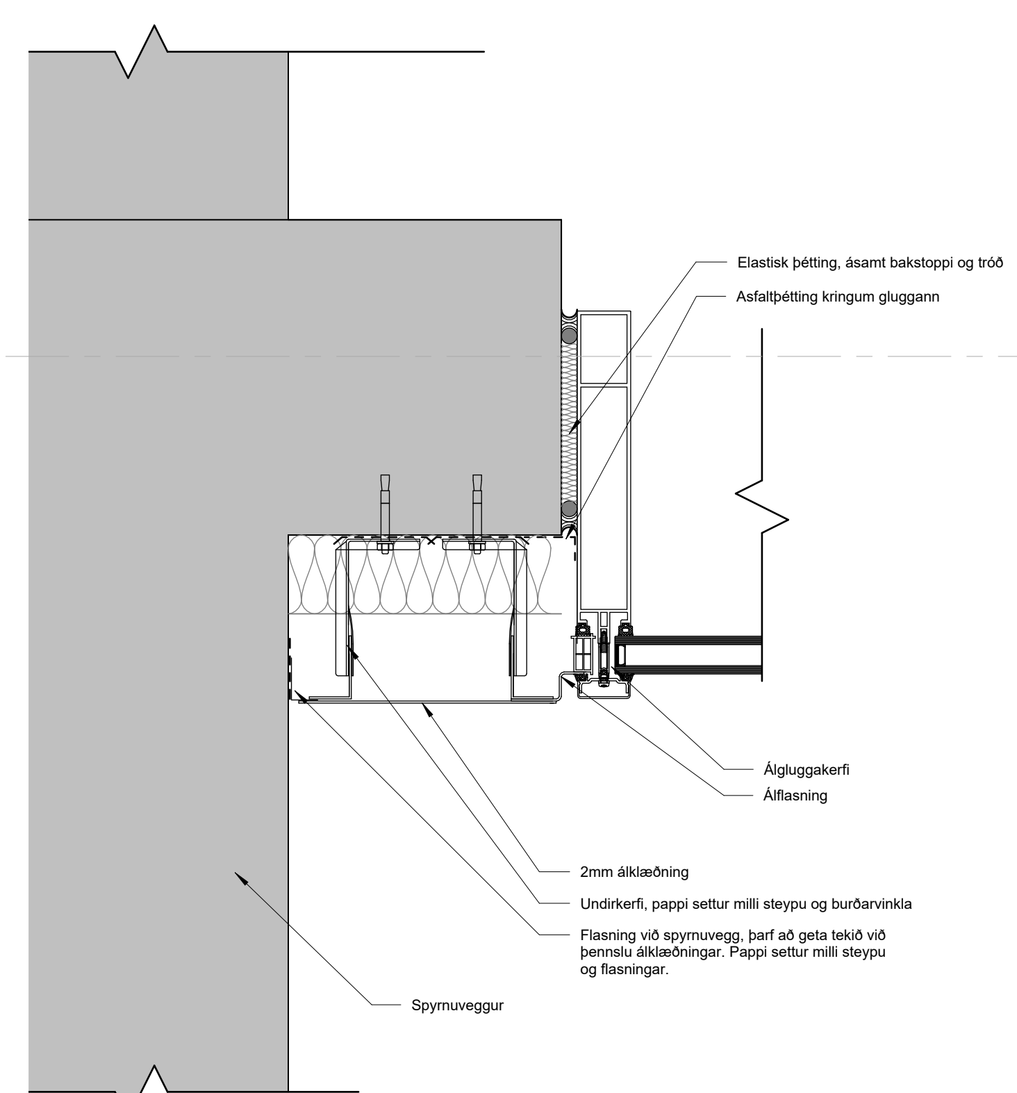
7 Frágangur við spyrnur 1:5
