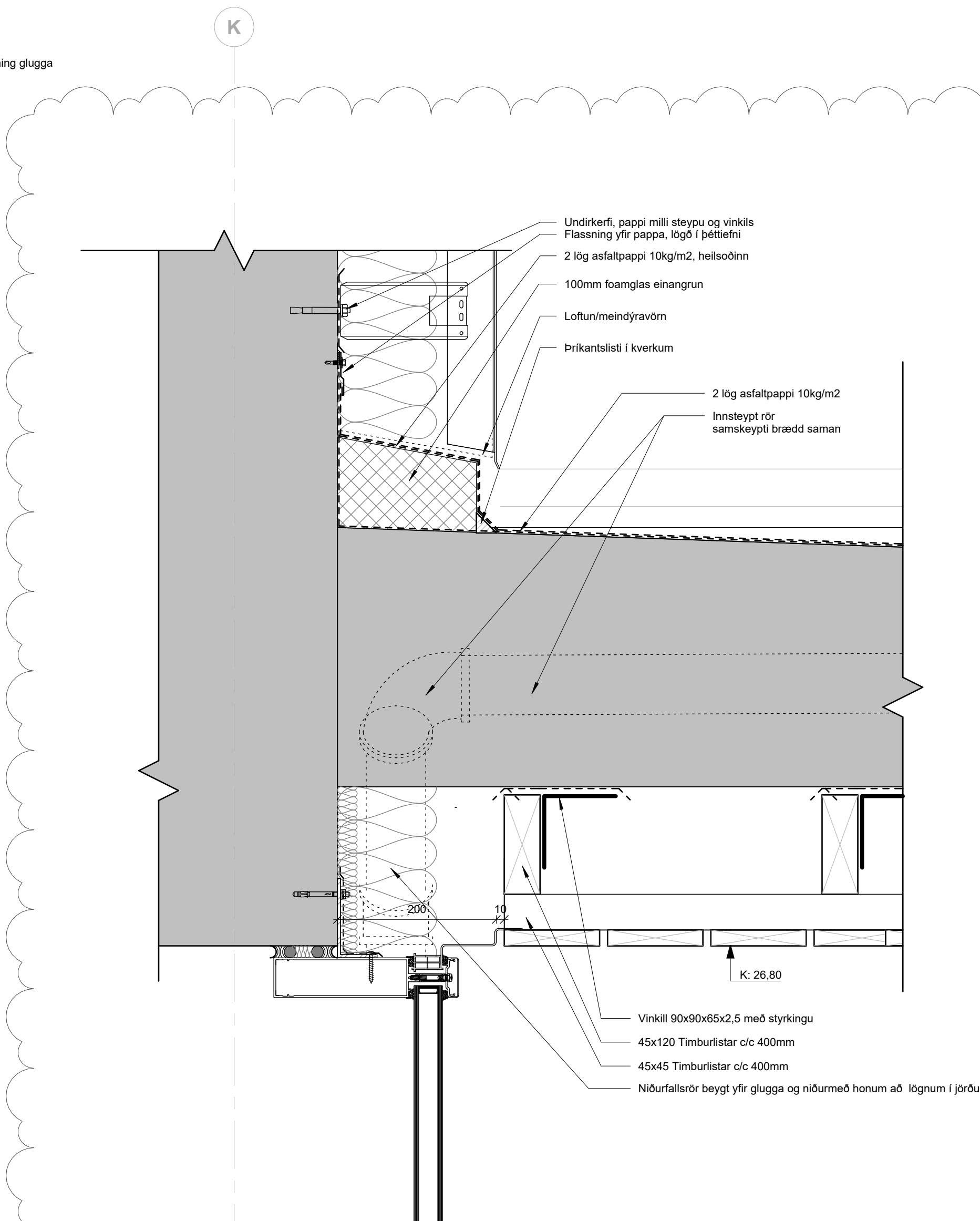
3 Frágangur við skyggni 1 : 5
