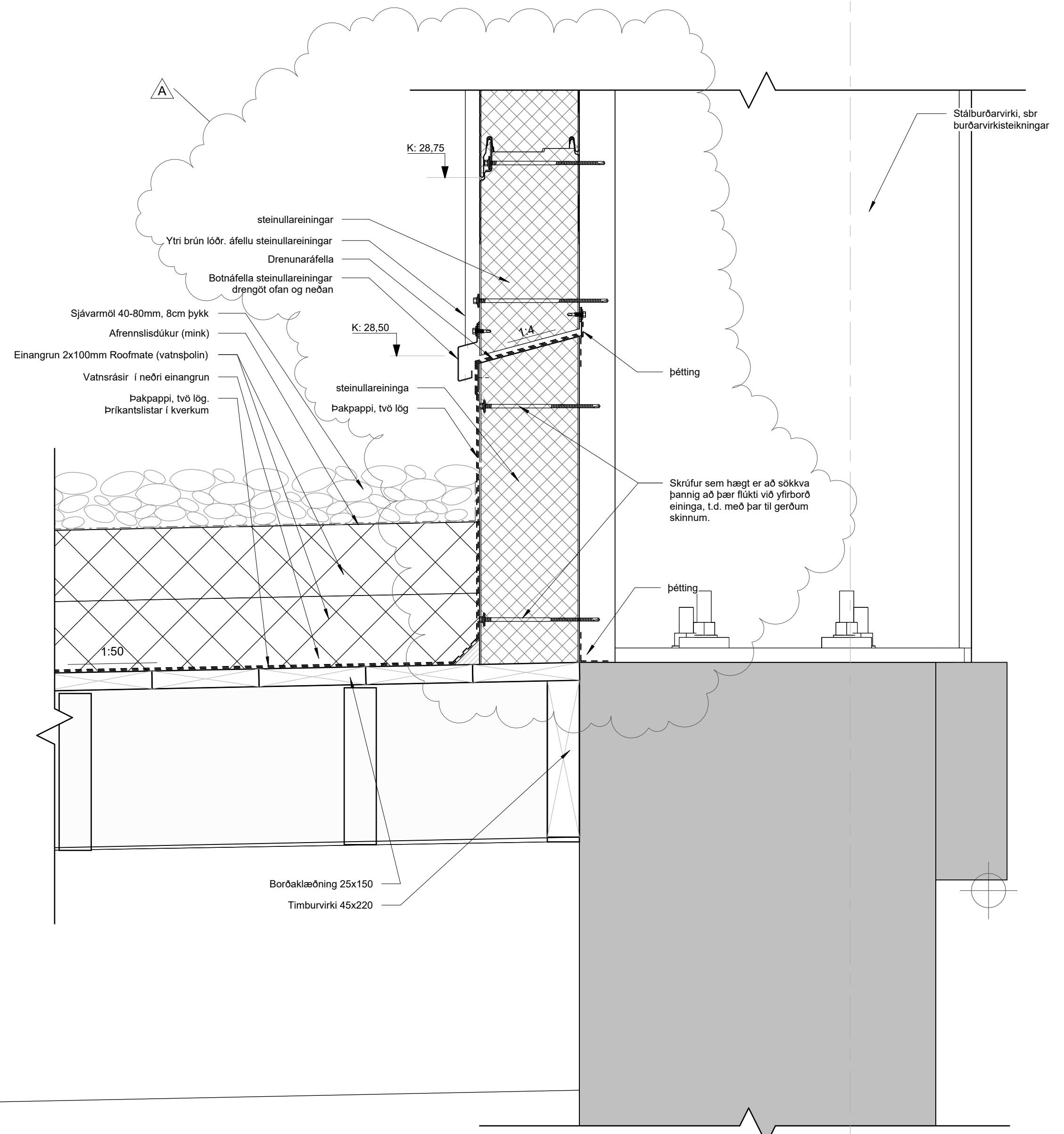
2 Viðsnúid þak, efri, timburþak 1 : 5
