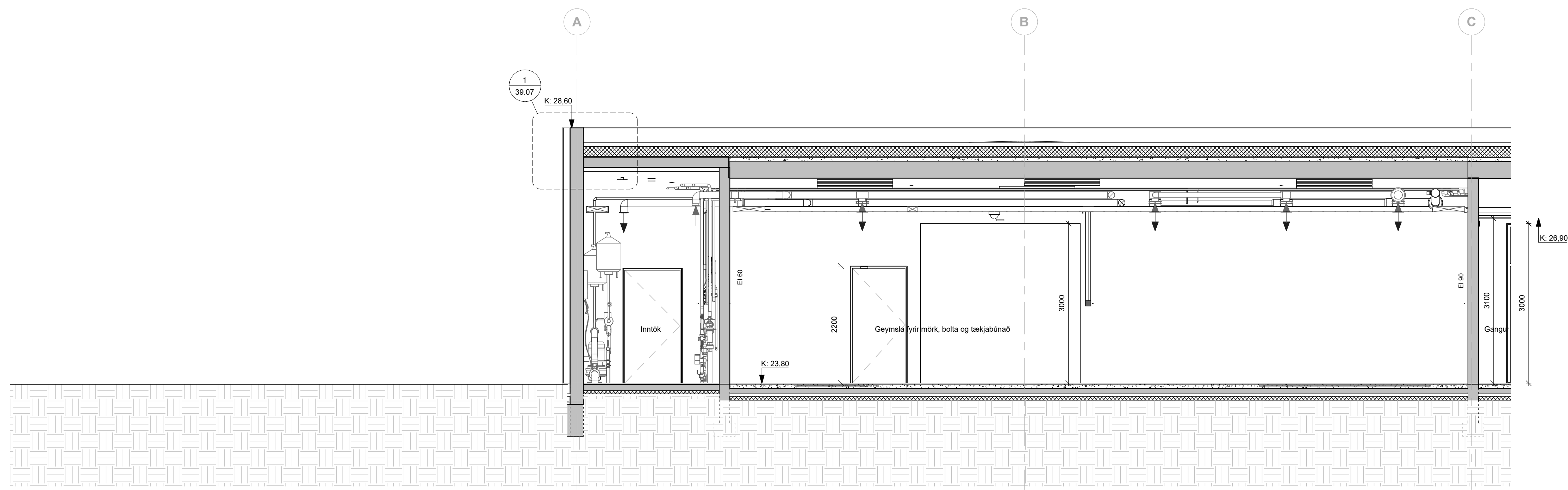
1 20-2-S - Hluti 1 1 : 50
