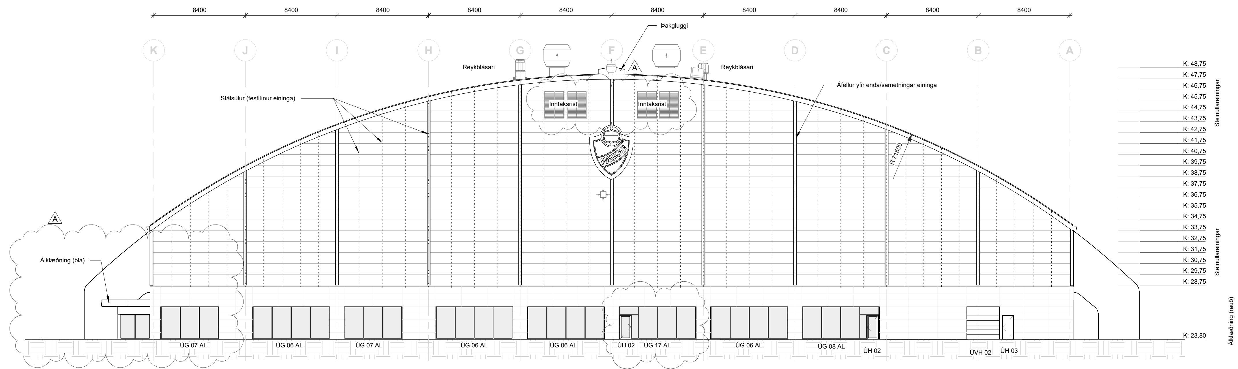
1 Suður - Útlit 1 : 200
