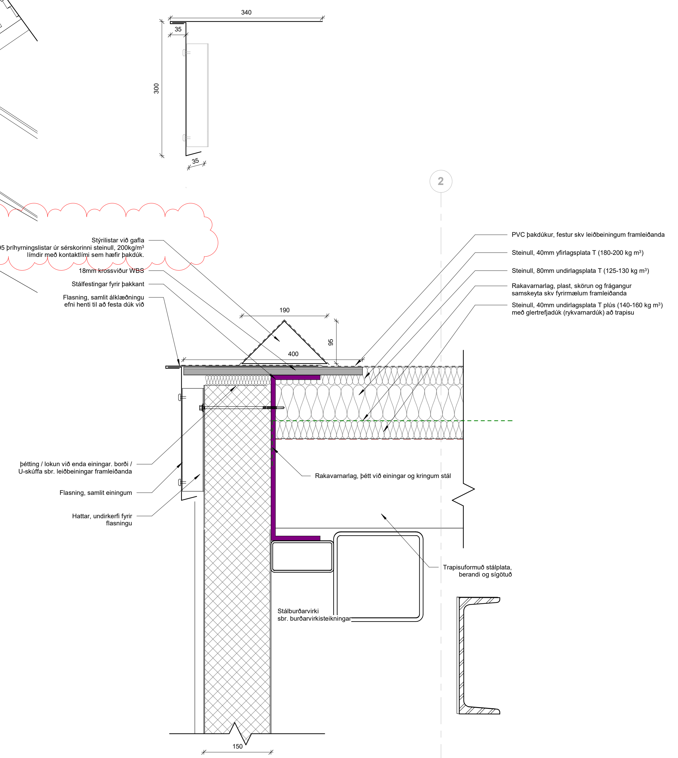
2 Þak, salur, þakkantur 1 : 5
