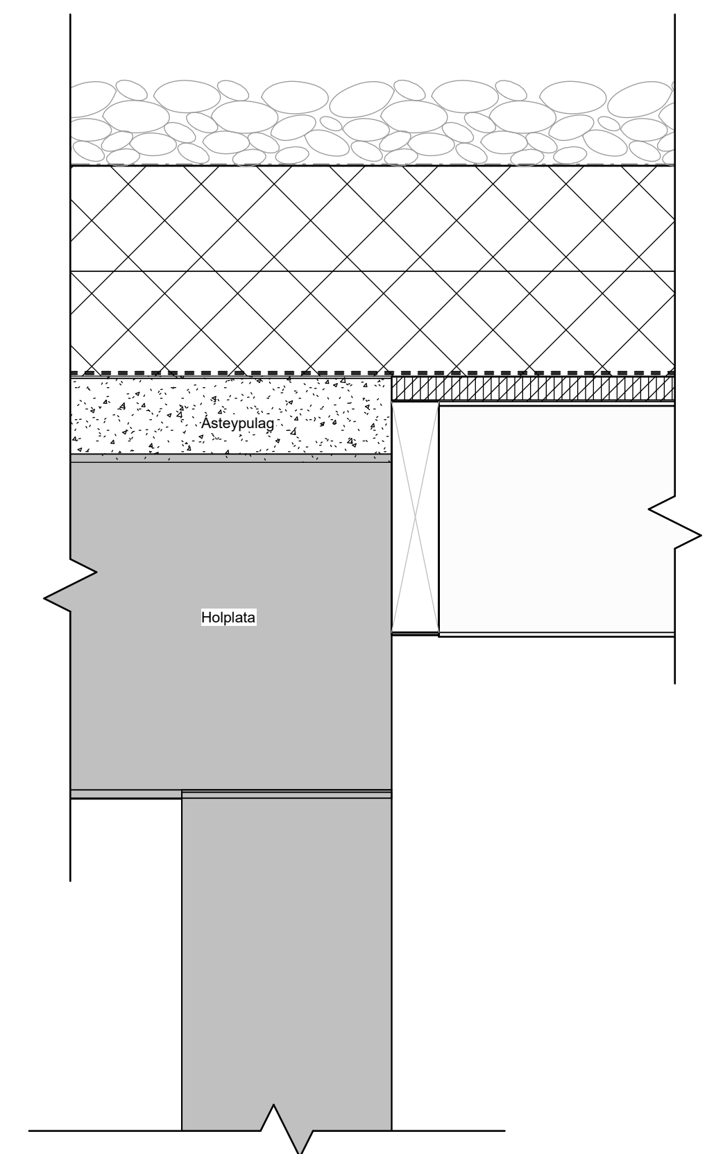
1 Timburþak 1 : 5
