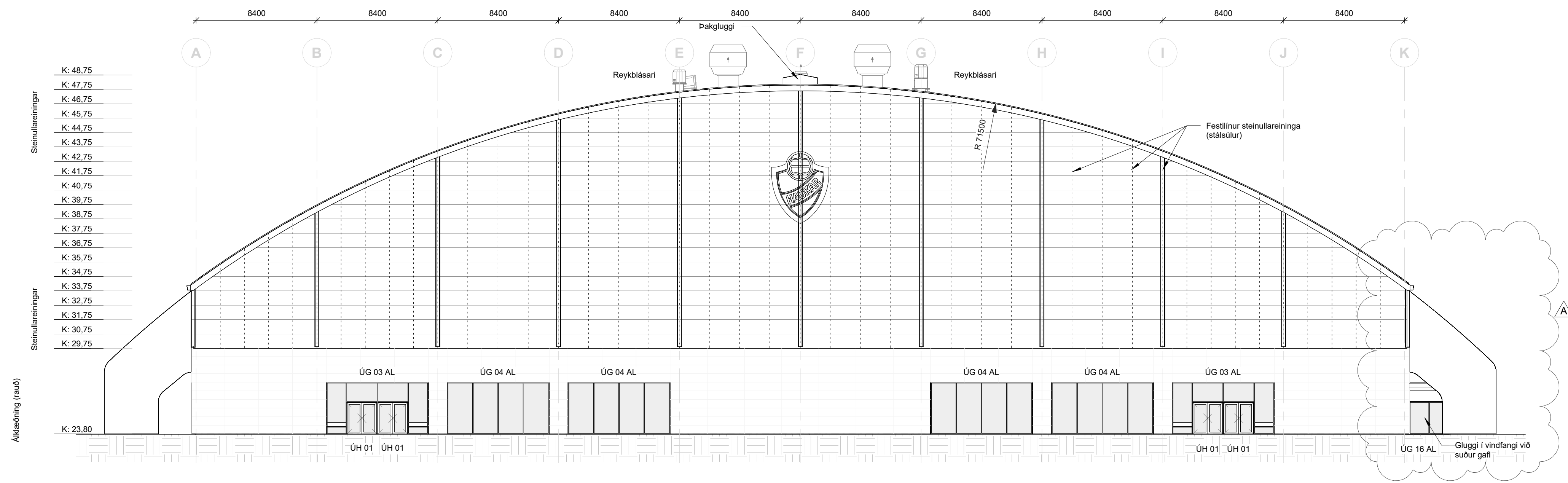
1 Norður - Útlit 1 : 200
