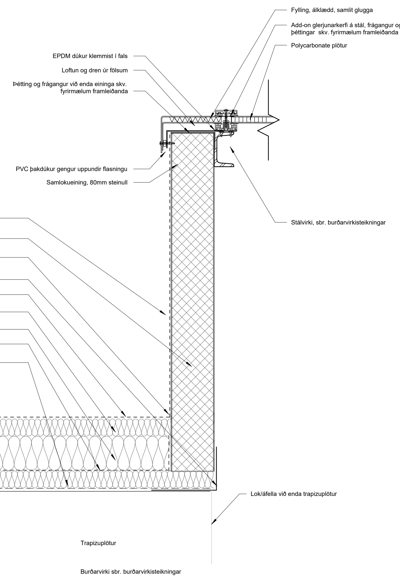
2 Þakgluggi, langsnið 1 : 5
