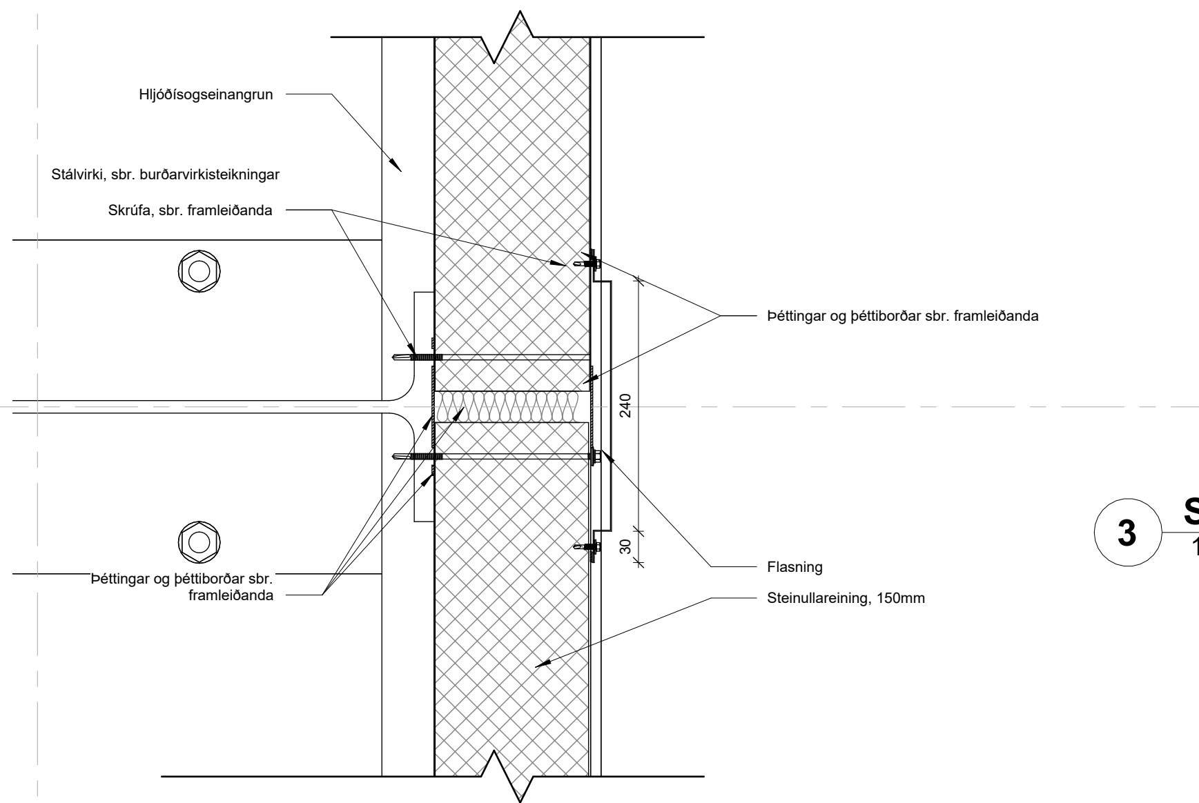
2 Steinullareiningar, samsetning 1 : 5
