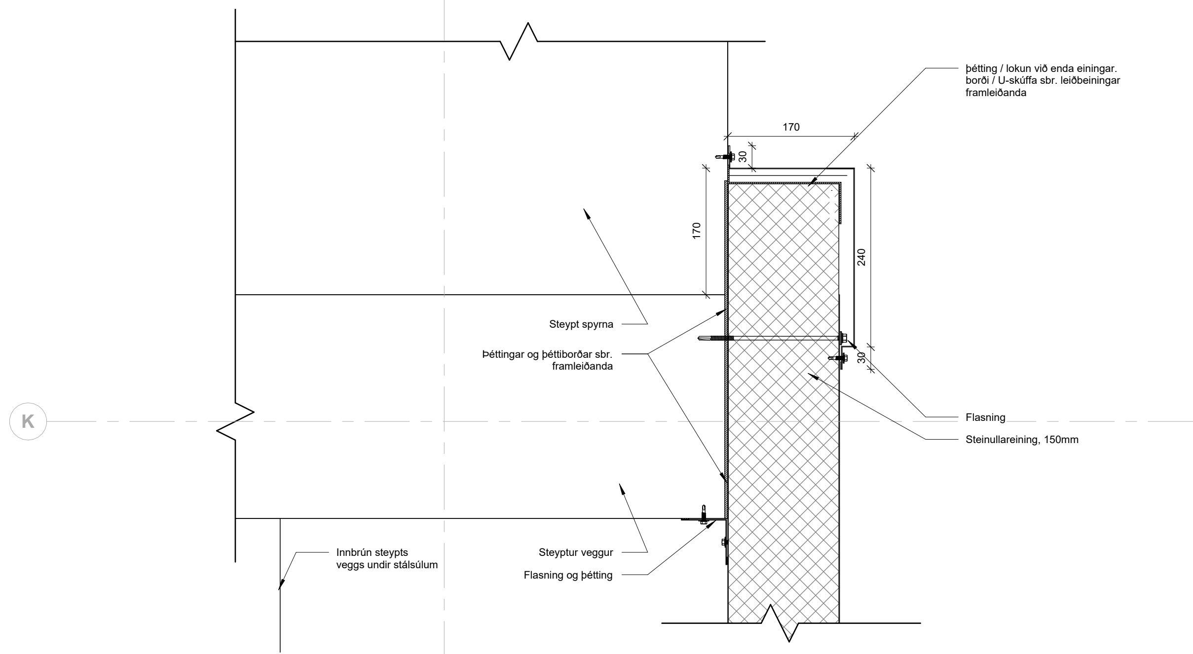
1 Steinullareiningar, horn 1 : 5
