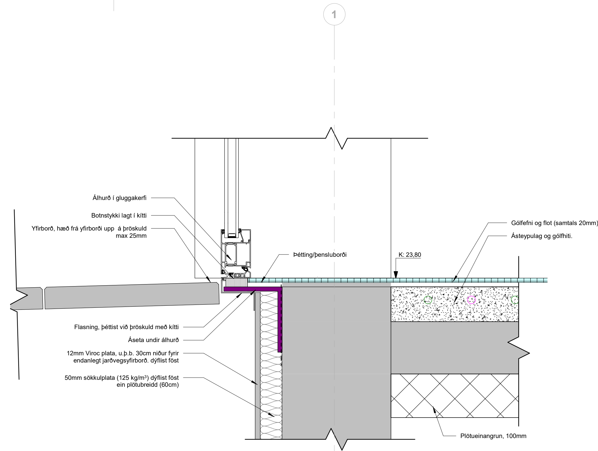
4 Sökkull, álhurð 1 : 5
