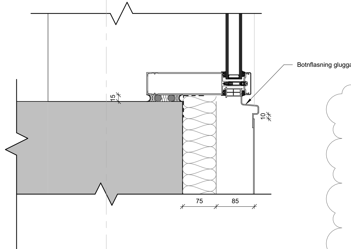
1 Álklaðning, salur, álguggi, ofan og neðan 1 : 5
