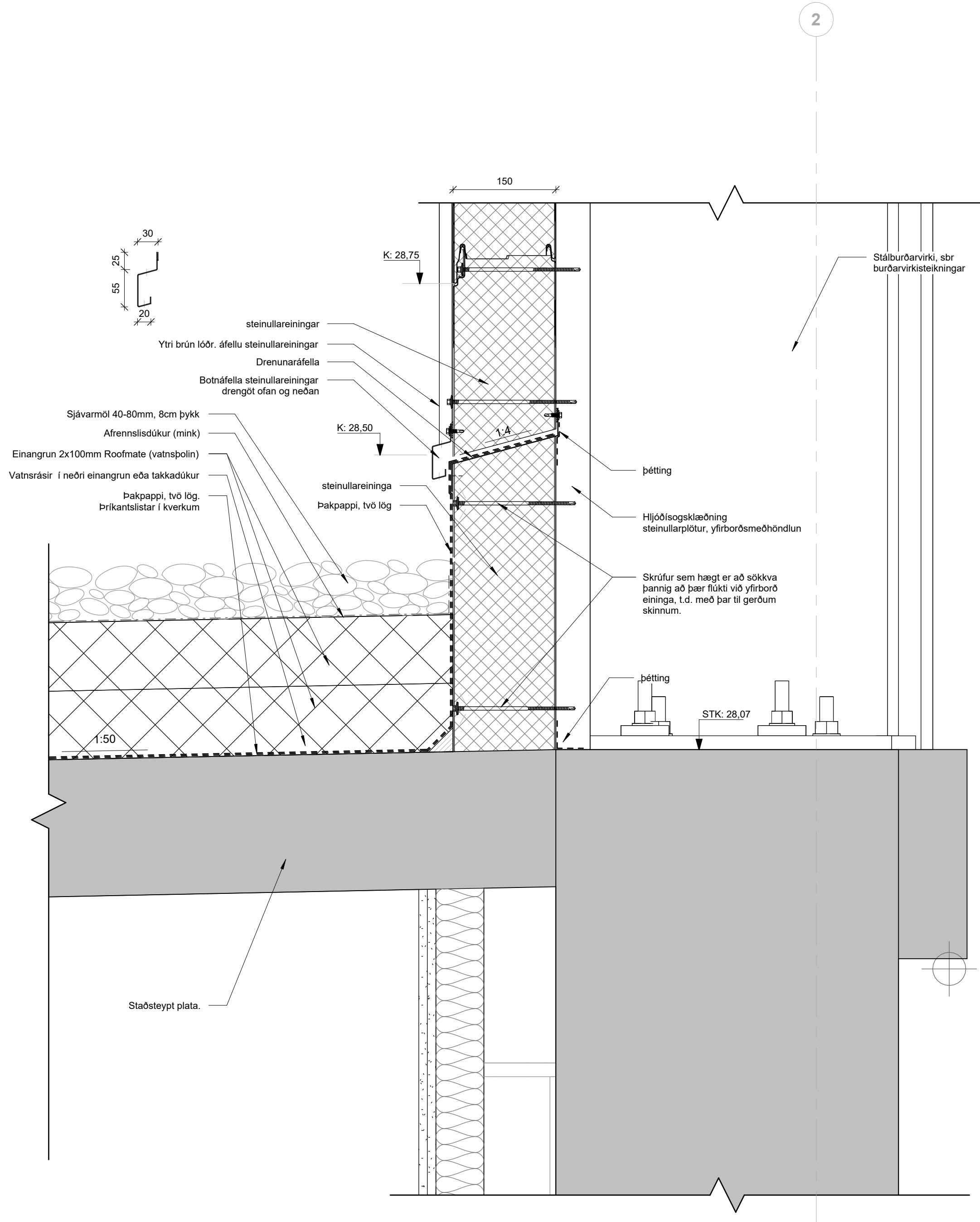
2 Viðsnúid þak, efri, Staðsteypt plata 1 : 5
